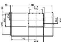
MMF-AP1445DHP-VA/VB, MMF-AP1925DHP-VA/VB
