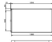
MMF-AP1445HP-VA/VB, MMF-AP1925HP-VA/VB
