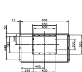
MMF-AP0725DHP-VA/VB, MMF-AP0965DHP-VA/VB
