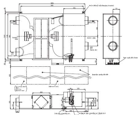
MMD-VN502HEX1E
